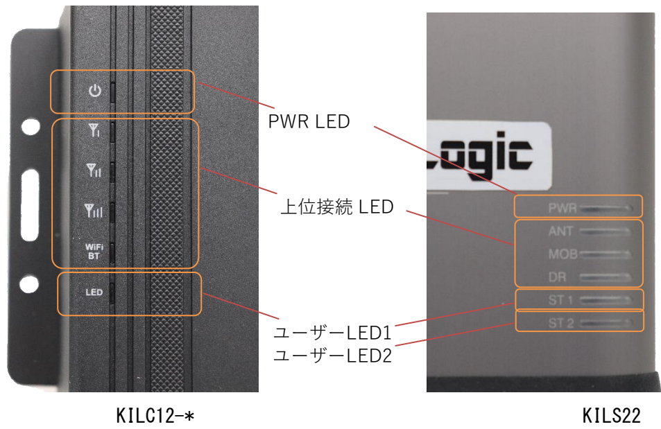
図 10 LED 配置
