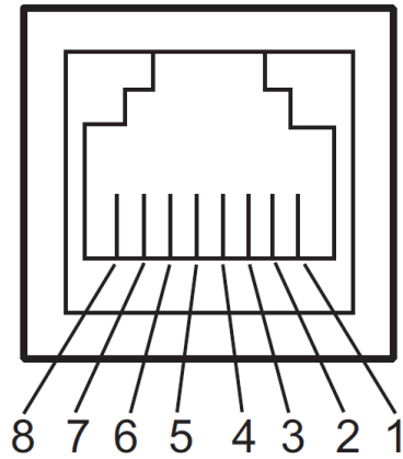
図 7 コネクタ
