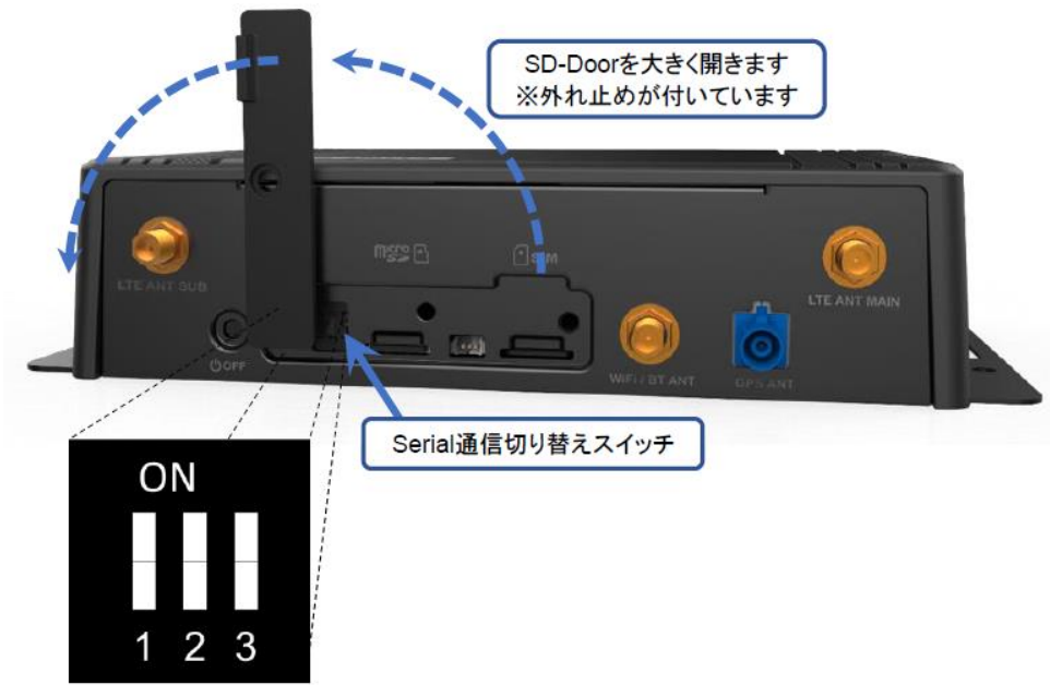
図 8 SW
