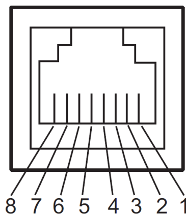
図 9 コネクタ
