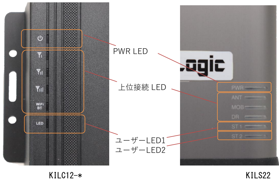
図 11 LED 配置
