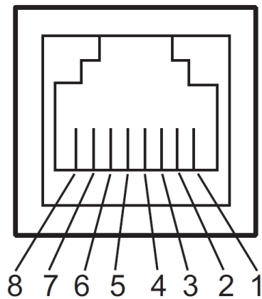
図 8 コネクタ
