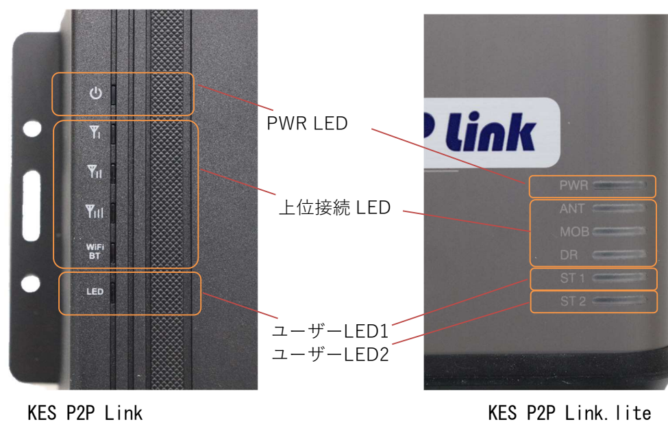
図 9 LED 配置
