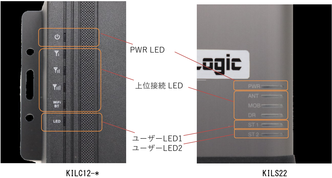
図 11 LED 配置
