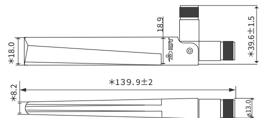
【CoralEdge用アンテナ】
