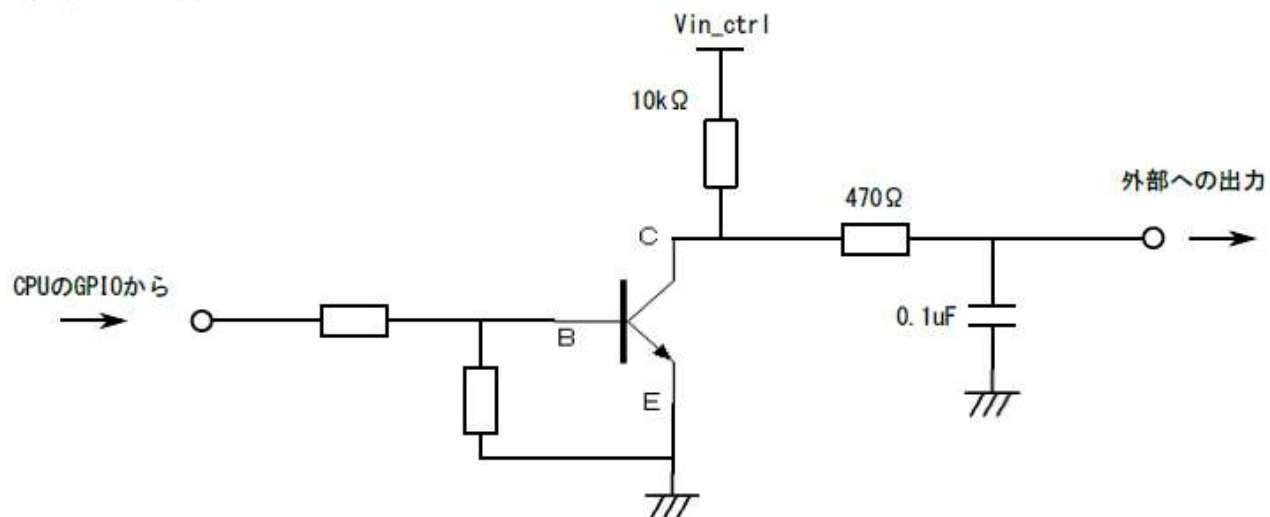
DO回路ブロック図
