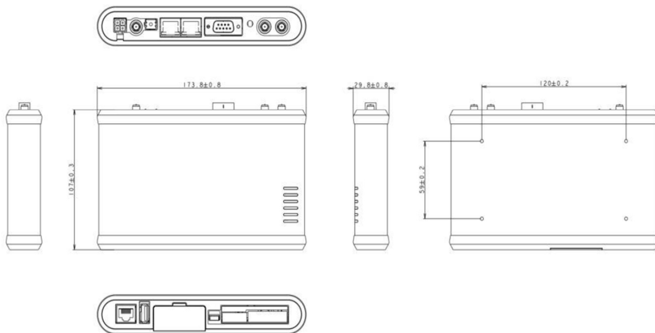
図 5 KILS22 外形
