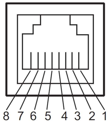
図 10 コネクタ
