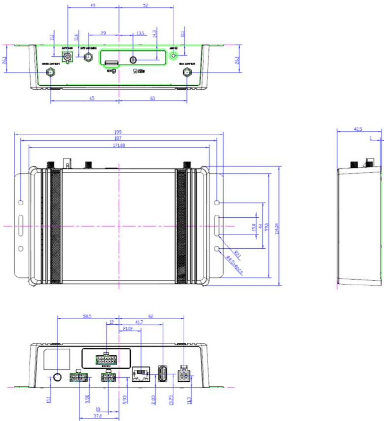
図 4 KILC12-*外形
