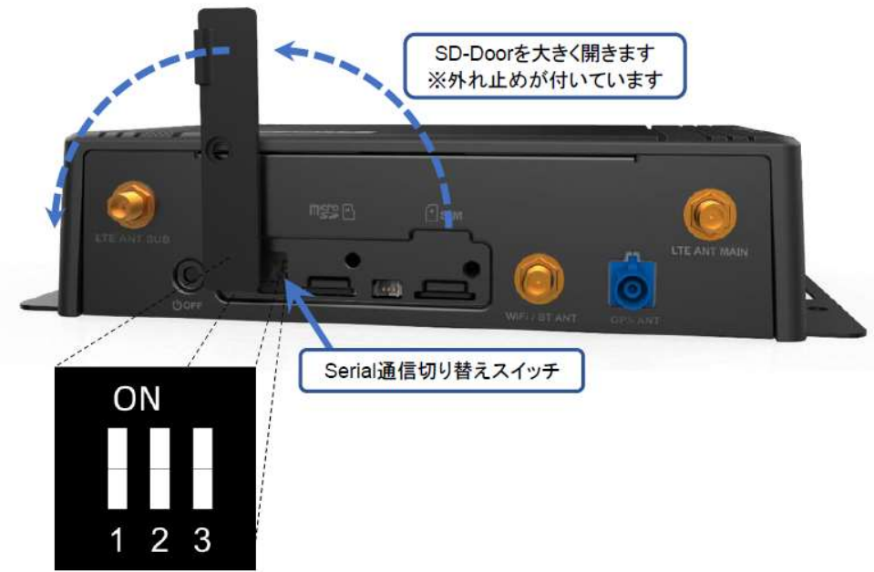
図 9 SW
