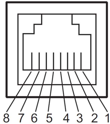
図 8 コネクタ
