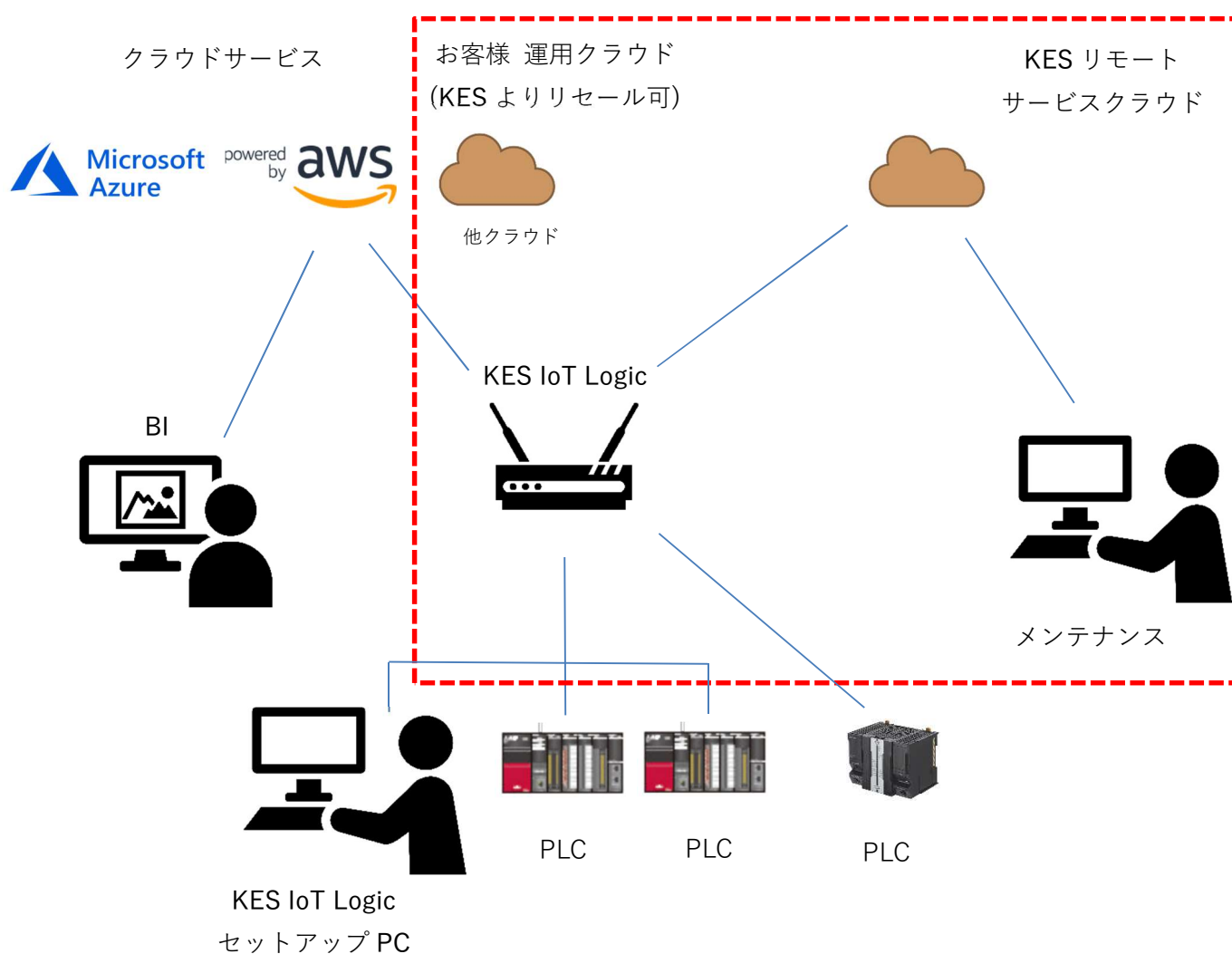
図 15 システム構成例
