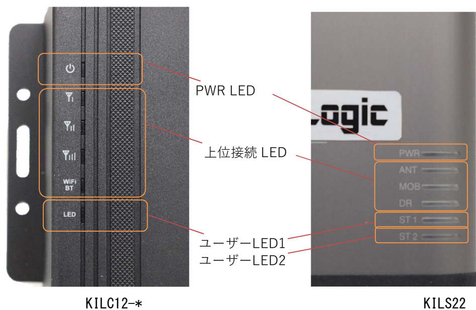
図 11 LED 配置
